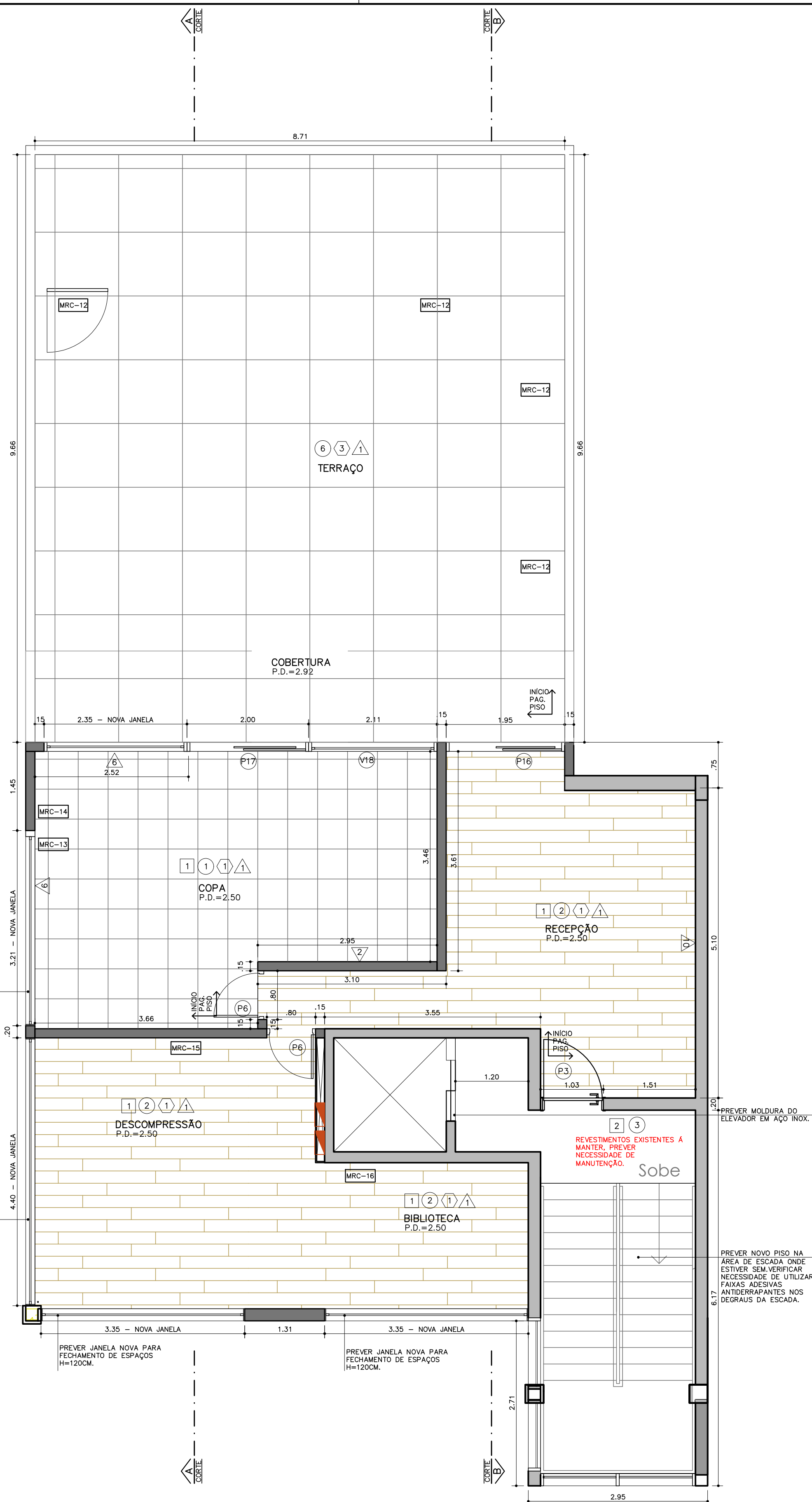
PLANTA DE ARQUITETURA – TERRAÇO ESCALA 1:50
