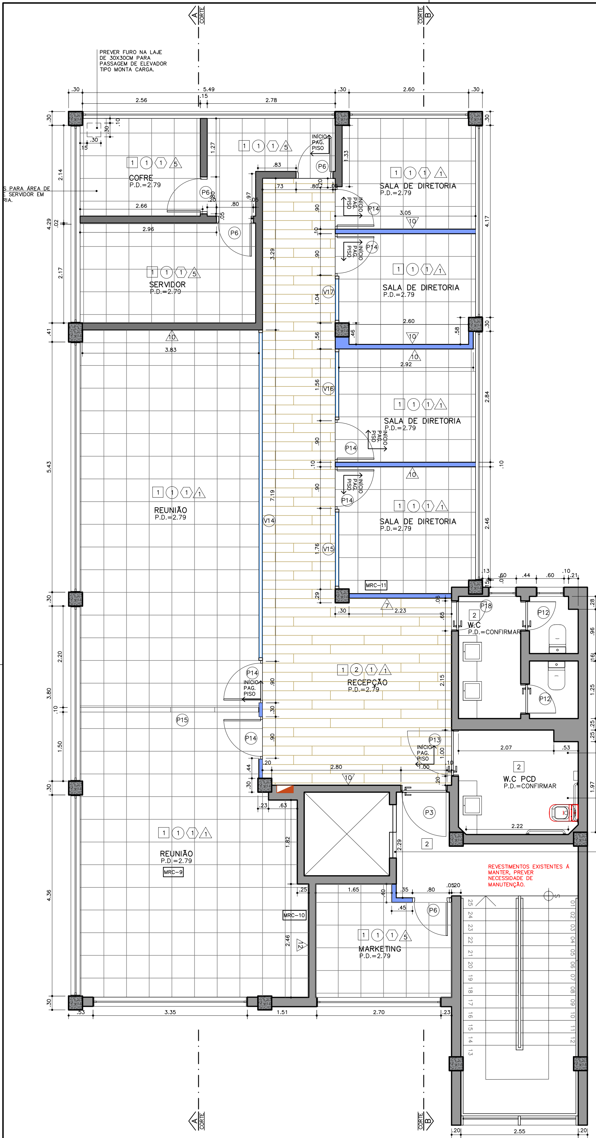
PLANTA DE ARQUITETURA – 1º PAVIMENTO ESCALA 1:50
